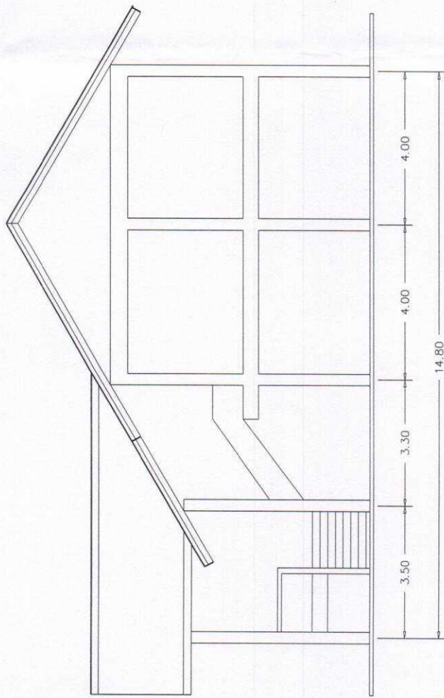
รูปด้านข้าง 1:100
