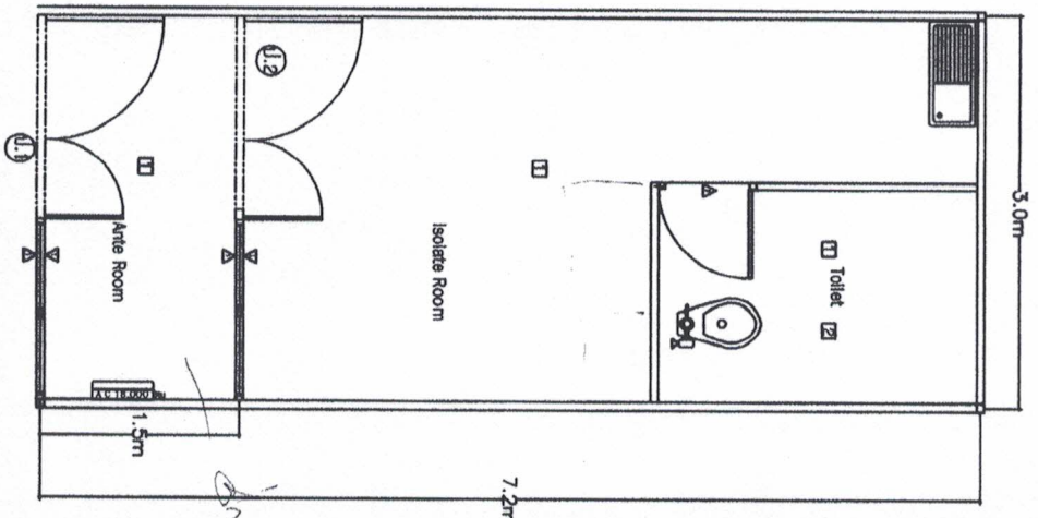
แผนห้องแยกโรค
