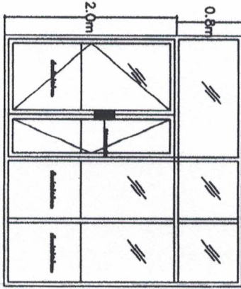
หน้าต่าง ประตู
